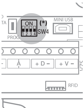
Switch SW4
